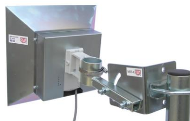
VBZ3 + konzolka MK5-K
