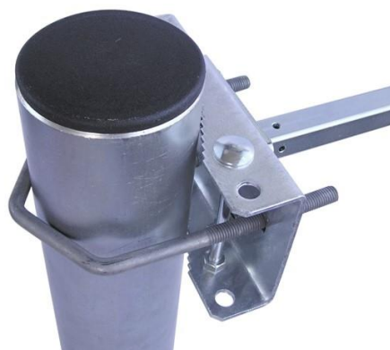
montáž na trubku s \varnothing 90mm
