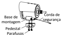
Figura 1-8 Fixação da câmara ao pedestal
