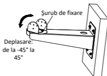
Figura 1-9 Ajustarea poziției de deplasare
