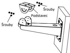
Obrázek 1-7 Demontáž podstavce
