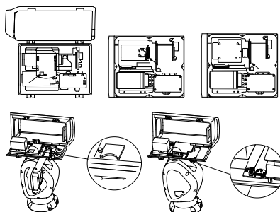
Figura 2-9 Slot per schede di memoria di diversi modelli
