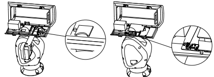
Abbildung 2-9 Speicherkartensteckplätze verschiedener Modelle
