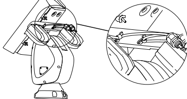
Obrázok 2-4 Pripevnite káble k IR držiaku
