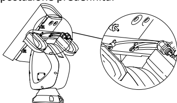
Figura 2-4 Fissare i cavi alla staffa IR
