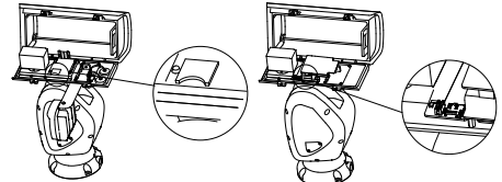
Ábra 2-9 Memóriakártya-nyílások különböző típusokon
