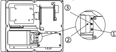
Abbildung 2-12 Laser einstellen (Typ IV der Serie DY9)
