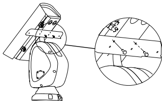
Obrázok 2-2 Pripevnite IR držiak
