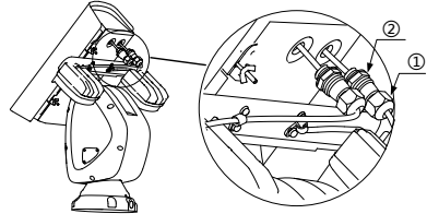
Imagen 2-5 Guíe los cables
