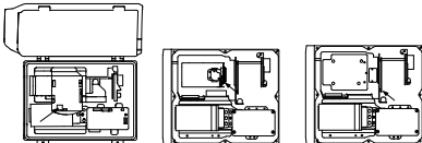
Imagen 2-8 Abra la cubierta (y la pantalla solar)
