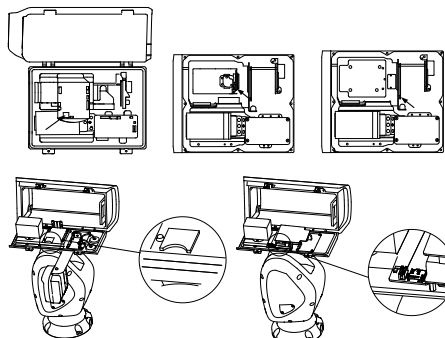
Figure 2-9 Logements de carte mémoire de différents modèles
