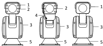
Рисунок 1-1 Система сетевого позиционирования серии DY7xxx
