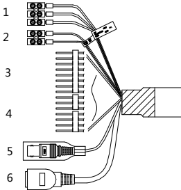
Figura 1-4 Cabluri I
