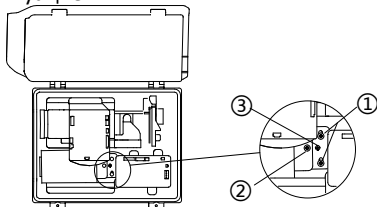
Рисунок 5-11 Регулировка лазера (тип III, серия DY9)
