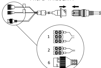
Рис. 1-5. Кабели II
