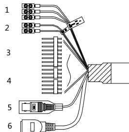
Rysunek 1-4 Przewody I
