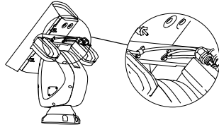
Рисунок 2-4 Прикріпіть кабелі до кронштейна модуля ІЧ-підсвічування
