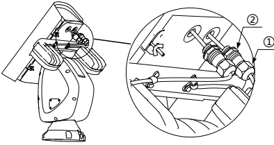
Şekil 2-5 Kabloları Yönlendirin
