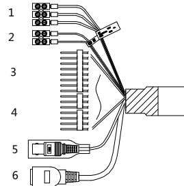
Şekil 1-4 Kablolar I
