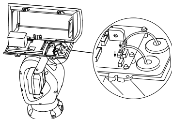
Obrázok 2-7 Pripojte káble
