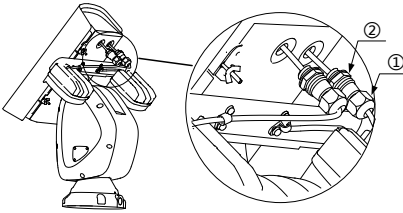
Abbildung 2-5 Kabel verlegen
