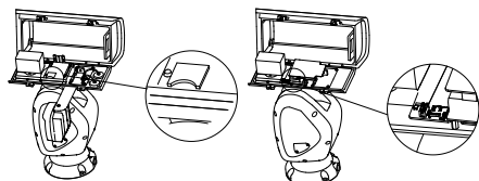
Figur 2-9 Pladser til hukommelseskort for forskellige modeller
