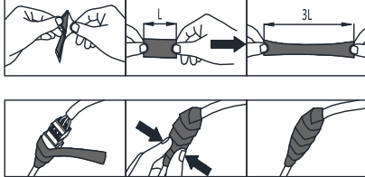
Şekil 2-14 Su geçirmez bantı kurun
