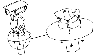
Figura 2-1 Fissare il sistema di posizionamento
