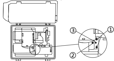
Şekil 2-11 Lazeri Ayarlayın (DY9 Serisinin Tip III'ü)
