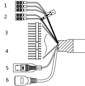
Figura 1-4. Cables I
