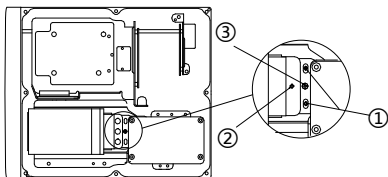
Рисунок 5-12 Регулировка лазера (тип IV, серия DY9)
