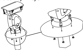
Rysunek 2-1 Mocowanie systemu pozycjonowania
