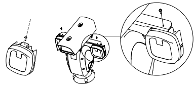
Abbildung 2-3 IR-Modul anschrauben
