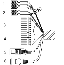
Figura 1-4 Cabos I
