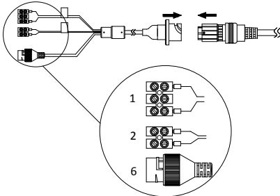
Abbildung 1-5 Kabel II Tabelle 1-2 Beschreibung der Kabel
