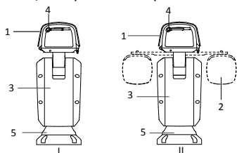
Рисунок 1-1 Система сетевого позиционирования серии DY7xxx
