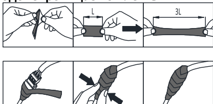
Рисунок 5-13 Установка водонепроницаемой оболочки
