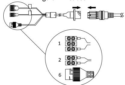
Figura 1-5 Cabos II
