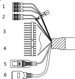
Рис. 1-4. Кабели I
