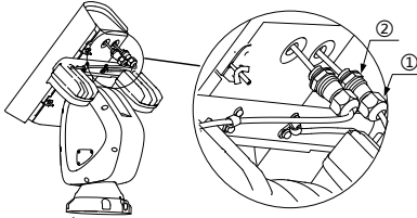
Ábra 2-5 A kábelek elvezetése
