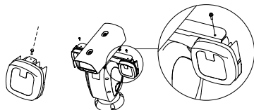
Rysunek 2-3 Mocowanie promiennika podczerwieni
