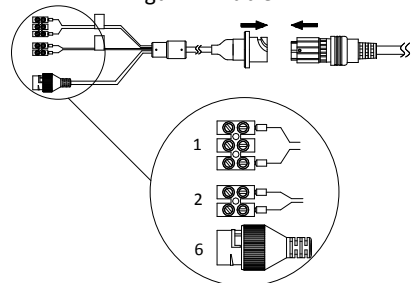
Figur 1-5 Kabler II Tabel 1-2 Kabelbeskrivelse
