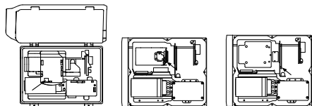
Figura 2-12 Ajustar o laser (Tipo IV da série DY9)
