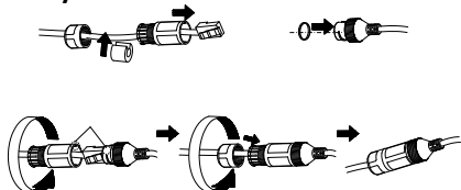
Ábra 2-13 A vízálló köpeny felhelyezése
