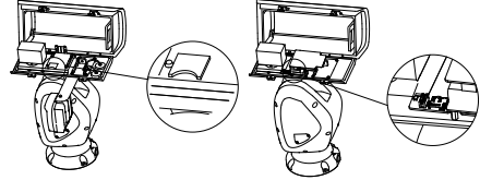
Şekil 2-9 Farklı Modellerin Hafıza Kartı Yuvaları
