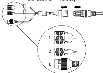
Obrázek 1-5 Kabely II Tabulka 1-2 Popis kabelů
