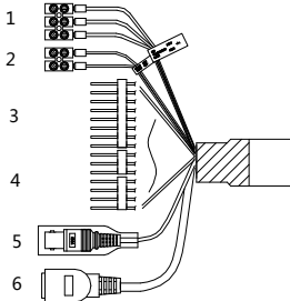
Afbeelding 1-4 Kabels I
