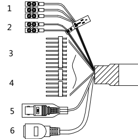
Рисунок 1-4. Кабелі I
