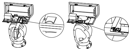
Figură 5-9 Sloturi pentru carduri de memorie ale diferitelor modele
