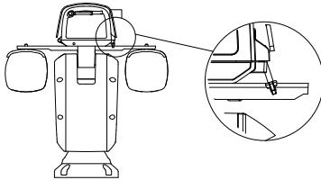
Abbildung 2-6 Gehäuse öffnen
