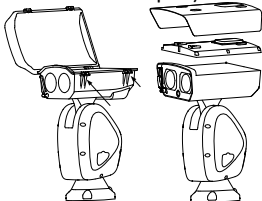
Рисунок 2-8 Відкрийте кришку (та сонцезахисний козирок)
