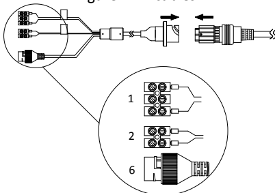
Figure 1-5 : câbles II
