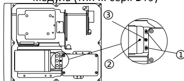
Рисунок 2-12 Відрегулюйте лазерний модуль (тип IV серії DY9)
