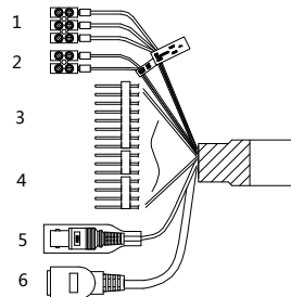
Gambar 1-4 Kabel I
