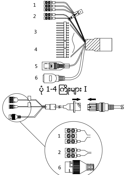
ပုံ 1-5 ကြိုးများ II
