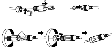
Figură 5-13 Instalați învelișul impermeabil al cablului de rețea
