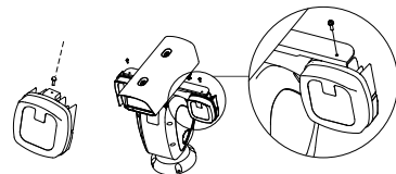
Figura 2-3 Fissare il modulo IR
