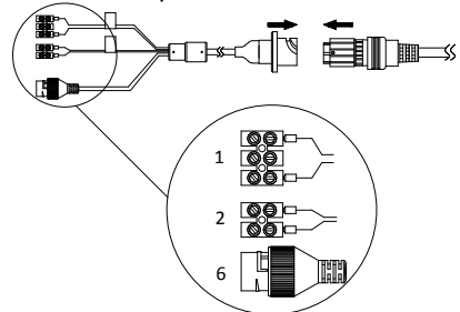
Рисунок 1-5. Кабелі II Таблиця 1-2 Опис кабелів
