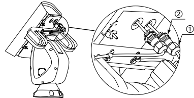
Рисунок 2-5 Прокладіть кабелі
