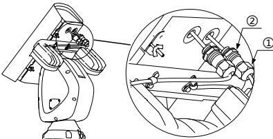
Figure 2-5 Acheminement des câbles
