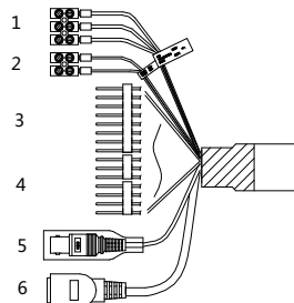
Obrázek 1-4 Kabely I
