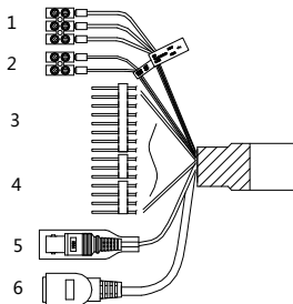
Obrázok 1-4 Káble I
