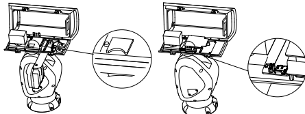
Rysunek 2-9 Gniazda karty pamięci w poszczególnych modelach
