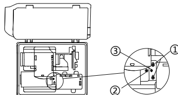
Obrázek 2-11 Upravení laseru (typ III řady DY9)
