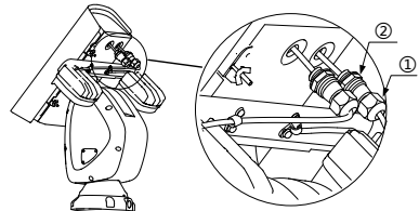
Figur 2-5 Træk kablerne
