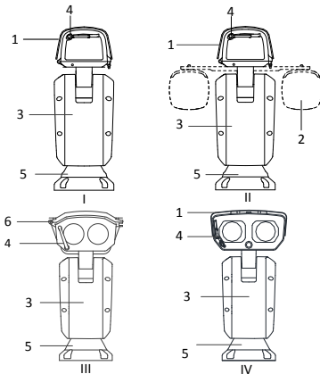
Figur 1-2 Netværkspositionerings-system i DY9xxx-serien
