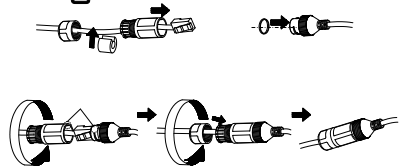
ပုံ 2-8 ရေစိုခံအပေါ်အုံ တပ်ဆင်ပါ
