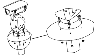
Figure 2-1 Fixation du système de positionnement
