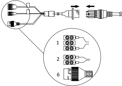
Şekil 1-5 Kablolar II Tablo 1-2 Kablo Açıklaması
