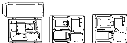
Figur 2-8 Åbn dækslet (og solskærm)
