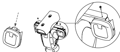
Ábra 2-3 Az IR-modul rögzítése
