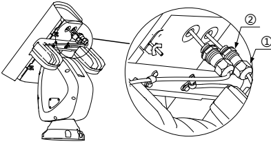
Gambar 2-5 Merutekan Kabel
