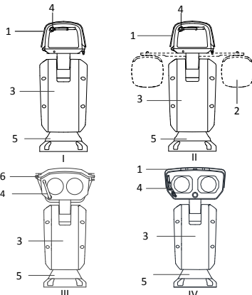
Figură 1-2 Sistem de poziționare în rețea Seria DY9xxx
