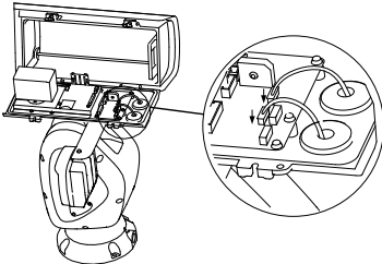
Abbildung 2-7 Kabel anschließen
