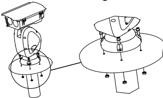
Abbildung 2-1 Positionierungssystem montieren
