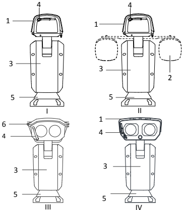
ပုံ 1-2 DY9xxx စီးရီးအလိုက်
