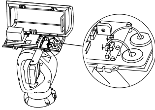
Rysunek 2-7 Podłączenie przewodów
