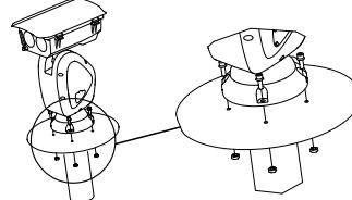
Figuur 2-1 Bevestig het positioneringssysteem
