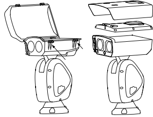
ပုံ 2-3 အဖုံး (နှင့် နေကာ) ကို ဖွင့်ပါ
