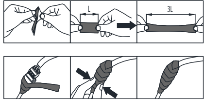
Abbildung 2-14 Wasserdichtes Klebeband installieren
