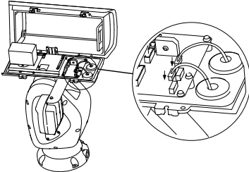
Şekil 2-7 Kabloları Bağlayın
