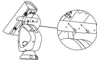
Figura 2-2 Fissare la staffa IR
