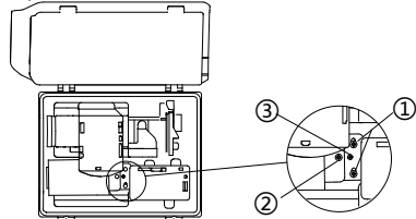
Rysunek 2-11 Regulacja lasera (typ III modeli DY9)
