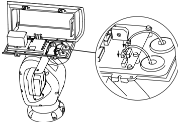
Gambar 2-7 Menghubungkan Kabel
