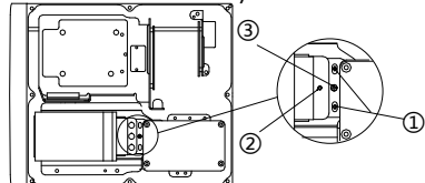
Rysunek 2-12 Regulacja lasera (typ IV modeli DY9)
