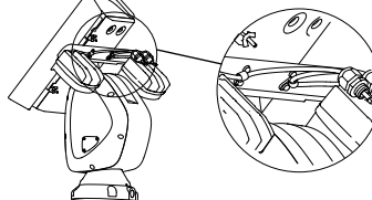
Ábra 2-4 A kábelek rögzítése az IR-modul rögzítőeleméhez
