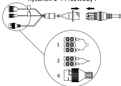
Rysunek 1-5 Przewody II Tabela 1-2 Opis przewodów
