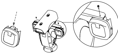
Imagen 2-3 Fije el módulo IR
