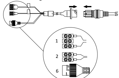
Figura 1-5. Cables II
