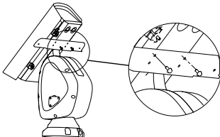
Figur 2-2 Fastgør IR-beslaget
