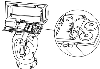
Рисунок 2-6 Відкрийте корпус
