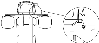
Obrázok 2-6 Otvorte kryt
