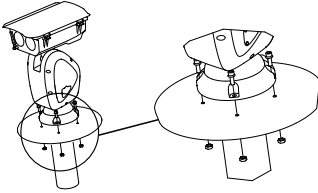
Imagen 2-1 Fije el sistema de posicionamiento
