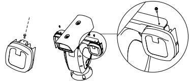
Figur 2-3 Fastgør IR-modulet 3. Fastgør spænderne til IR-beslaget med to M4 x 10 skruer.
