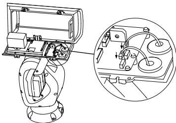
Рисунок 5-7 Подключение кабелей 2.3 Установка карты памяти (дополнительно)
