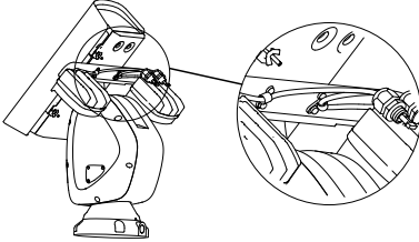
Figuur 2-4 Bevestig de kabels aan de IR-beugel
