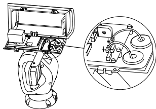
Figur 2-7 Tilslut kablerne
