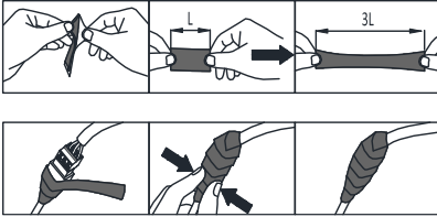
Figur 2-14 Installér den vandtætte tape
