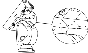
Abbildung 2-2 IR-Halterung montieren
