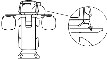
Şekil 2-6 Muhafazayı açın
