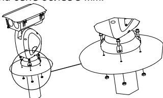
Рисунок 5-1 Монтаж системы позиционирования
