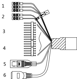
Ábra 1-4. Kábelek I
