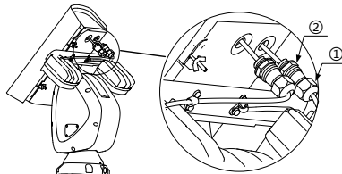
Рисунок 5-5 Прокладка кабелей
