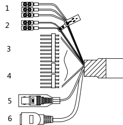
Abbildung 1-4 Kabel I
