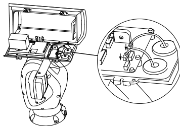
Figura 2-7 Collegare i cavi
