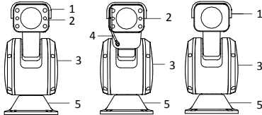
Figur 1-1 Netværkspositionerings-system i DY7xxx-serien
