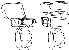
Obrázek 2-8 Otevření krytu (a sluneční clony) 3. Vložte paměťovou kartu do slotu pro paměťové karty podle konkrétní situace.
