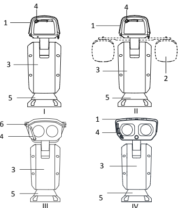
Obrázok 1-2 Sieťový pozičný systém série DY9xxx
