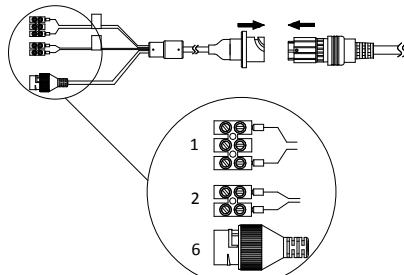
Obrázok 1-5 Káble II
