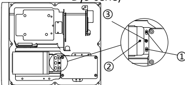
Figuur 2-12 Pas de laser aan (type IV van de DY9-serie)
