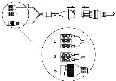
Ábra 1-5. Kábelek II 1-2. táblázat: A kábelek leírása
