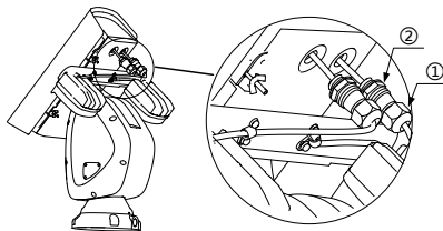
Obrázok 2-5 Umiestnite káble
