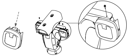
Figura 2-3 Fixar o Módulo IV 3. Fixe os grampos ao suporte IV com dois parafusos M4 x 10.
