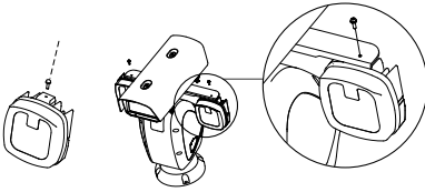
Figure 2-3 Fixation du module infrarouge
