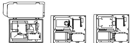
Figuur 2-8 Open het deksel (en het zonnenscherm)
