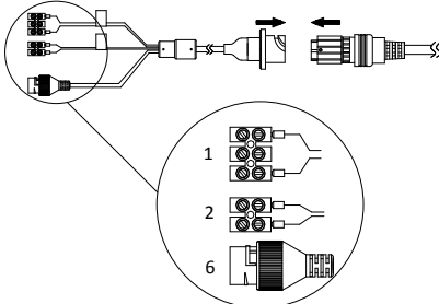
Figura 1-5 Cavi II Tabella 1-2 Cavi
