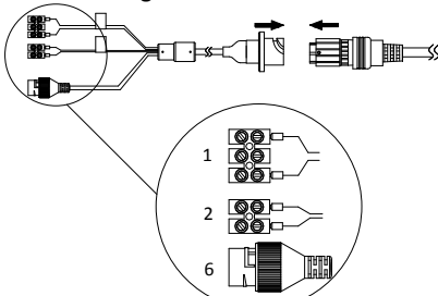
Figura 1-5 Cabluri II
