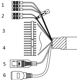
Figura 1-4 Cavi I
