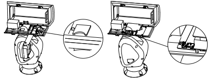
ပုံ 2-4 ပုံစံအမျိုးမျိုးရှိ မမ်ဗိုရီကတ်အပေါက်များ
